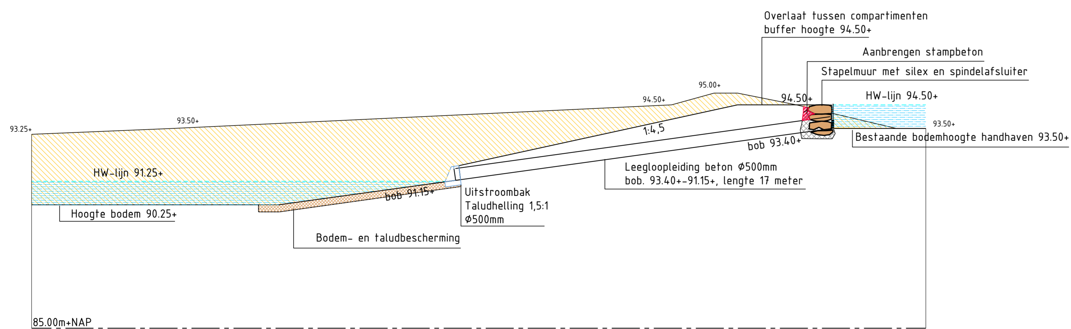
Profiel C-C buffer RESL21 Schaal 1:100
