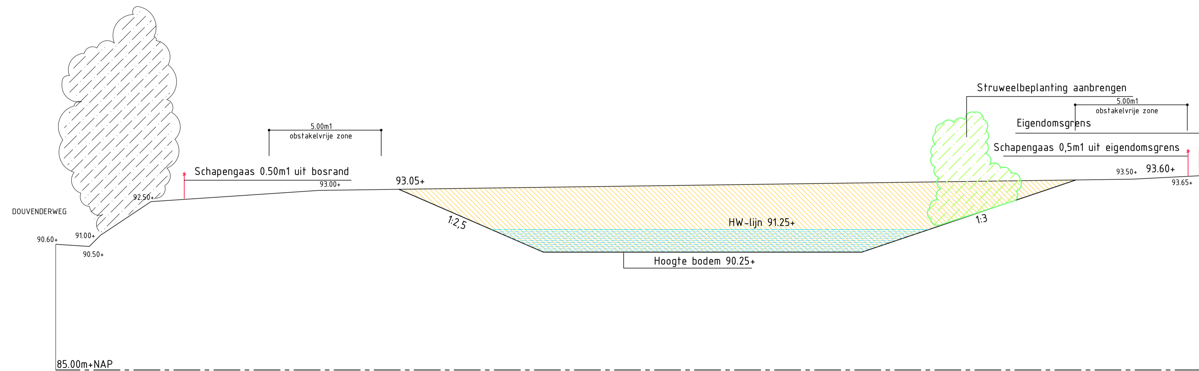
Profiel B-B buffer RESL21 Schaal 1:100
