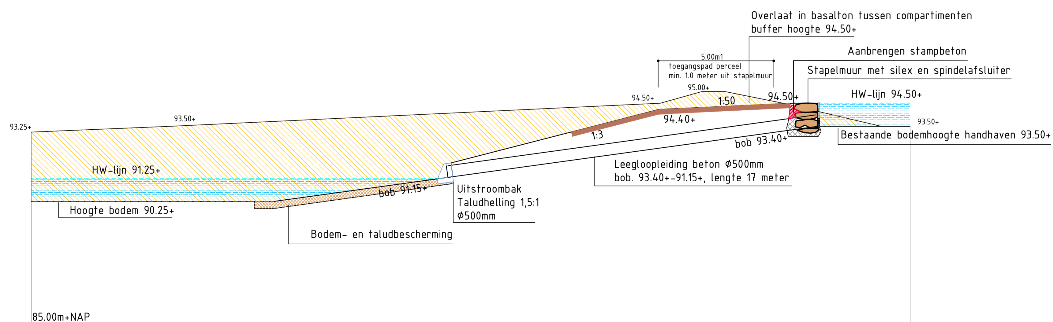
Profiel C-C buffer RESL21 Schaal 1:100
