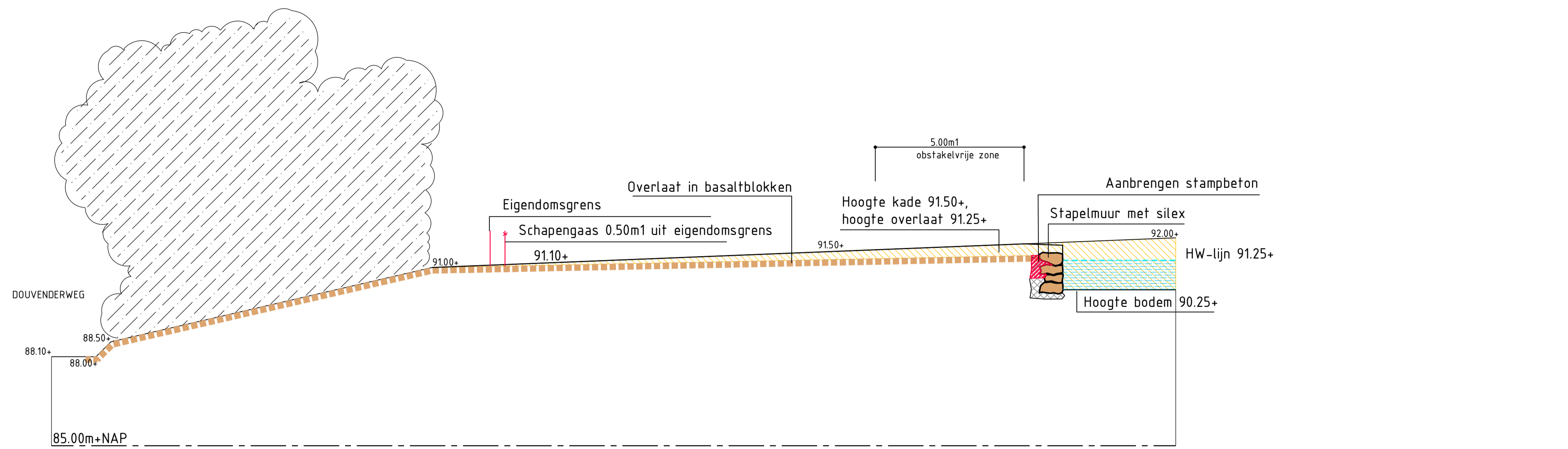
Profiel A-A buffer RESL21 Schaal 1:100
